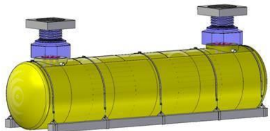
3D joonisel mahuti ankurdamine, TCI hoolduskaevud ja tänavaluugid.
